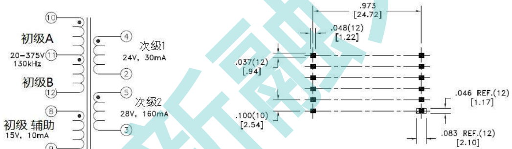
PCB封装图
